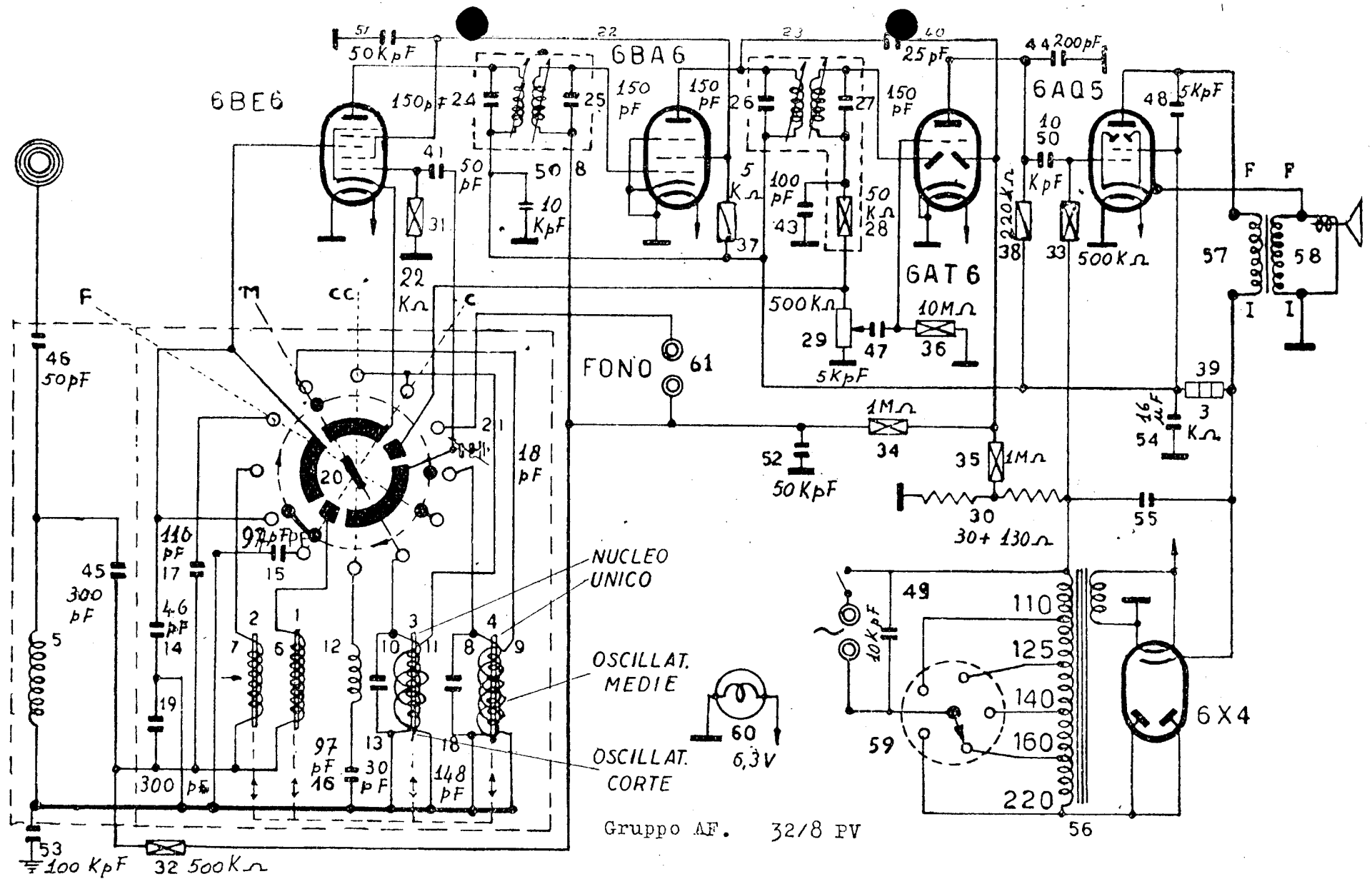
UNDA RADIO - Mod. R 53/24 B. Supereterodina a 3 gamme d'onda: 16-29; 29-52; 184-578 metri. Media frequenza 467 kc. Consumo: 28 watt; cc. 50 mA, ca. 175 mA. Potenza d'uscita 3 watt.
